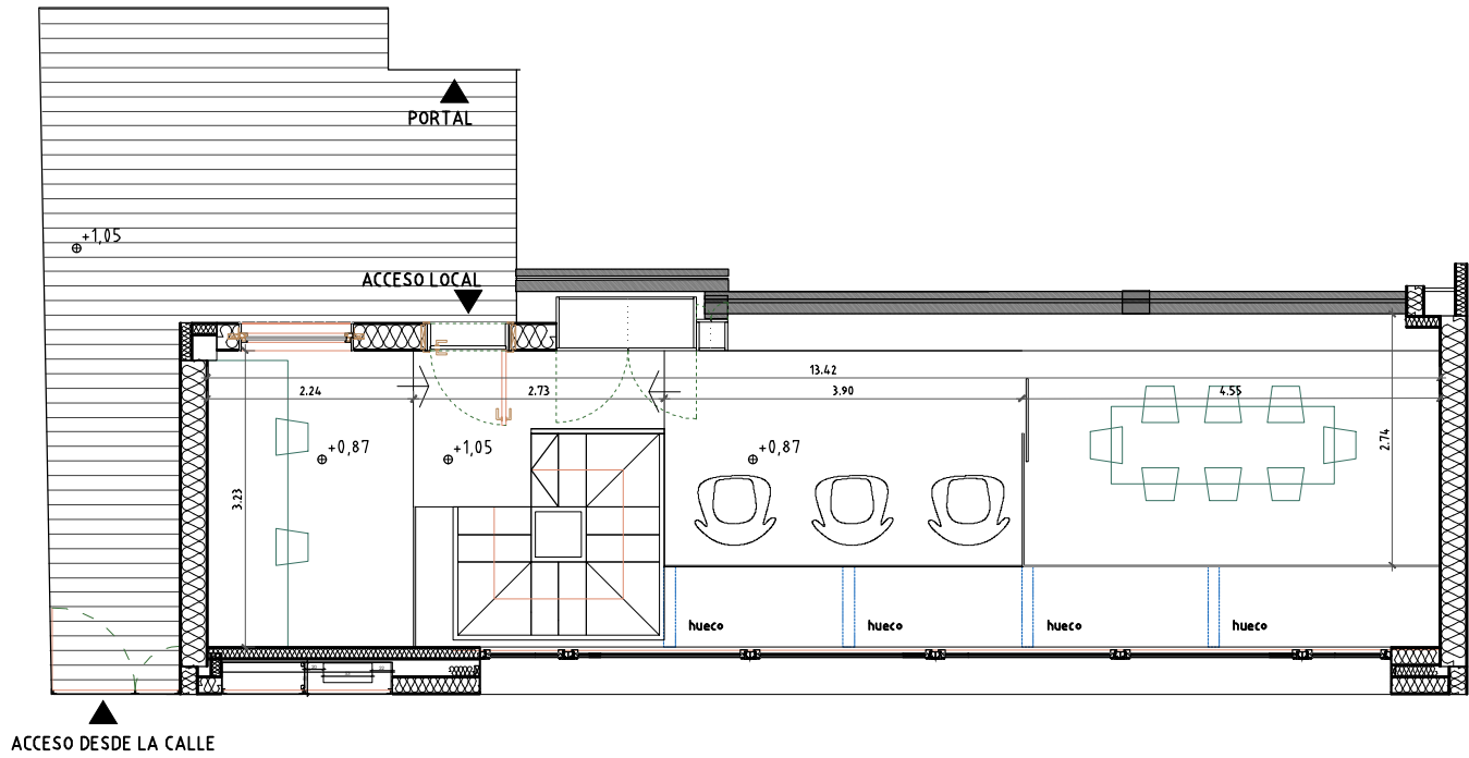
PLANTA INFERIOR SUPERFICIE ÚTIL: 35 m 2
