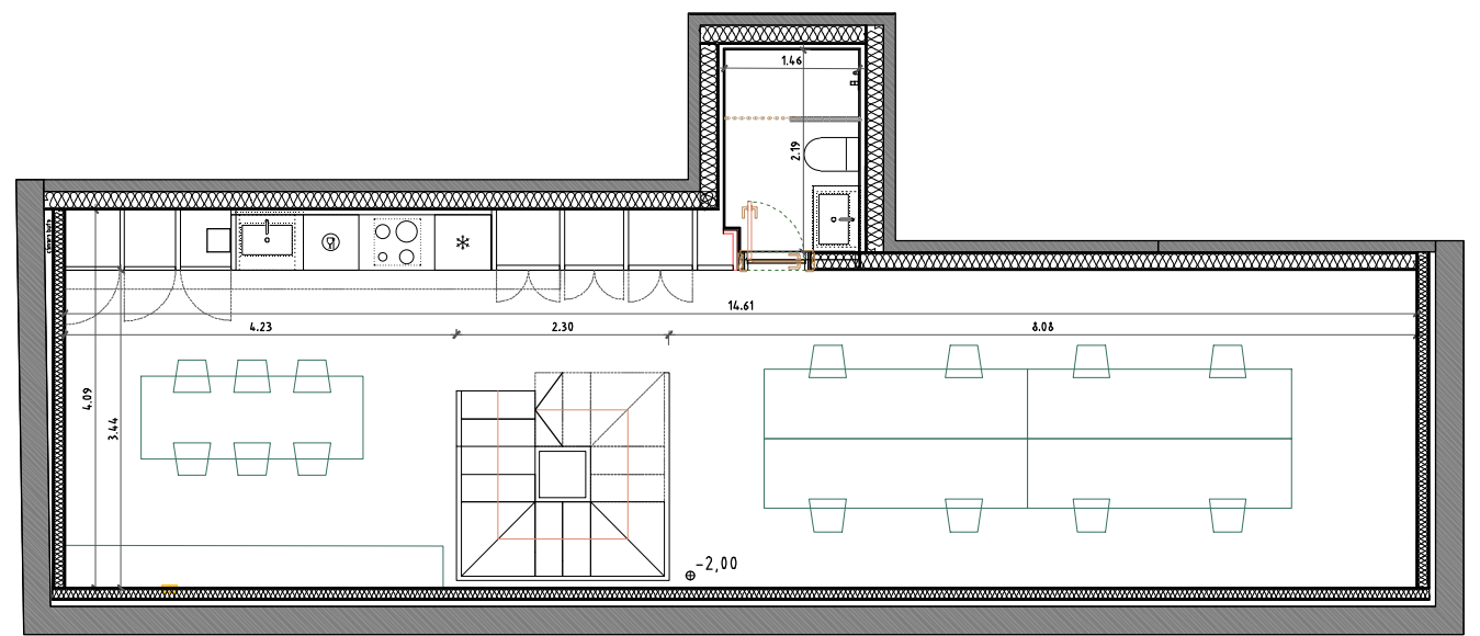
PLANTA INFERIOR SUPERFICIE ÚTIL: 58 m 2
